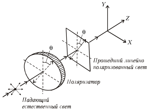
Рис. 3. Линейный поляризатор
